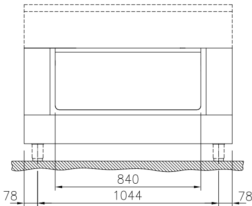
Zij aanzicht
